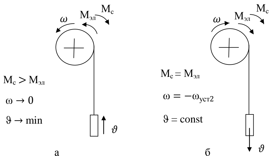
Рисунок 2.24 – Торможение ДПТ НВ в режиме противовключения:
