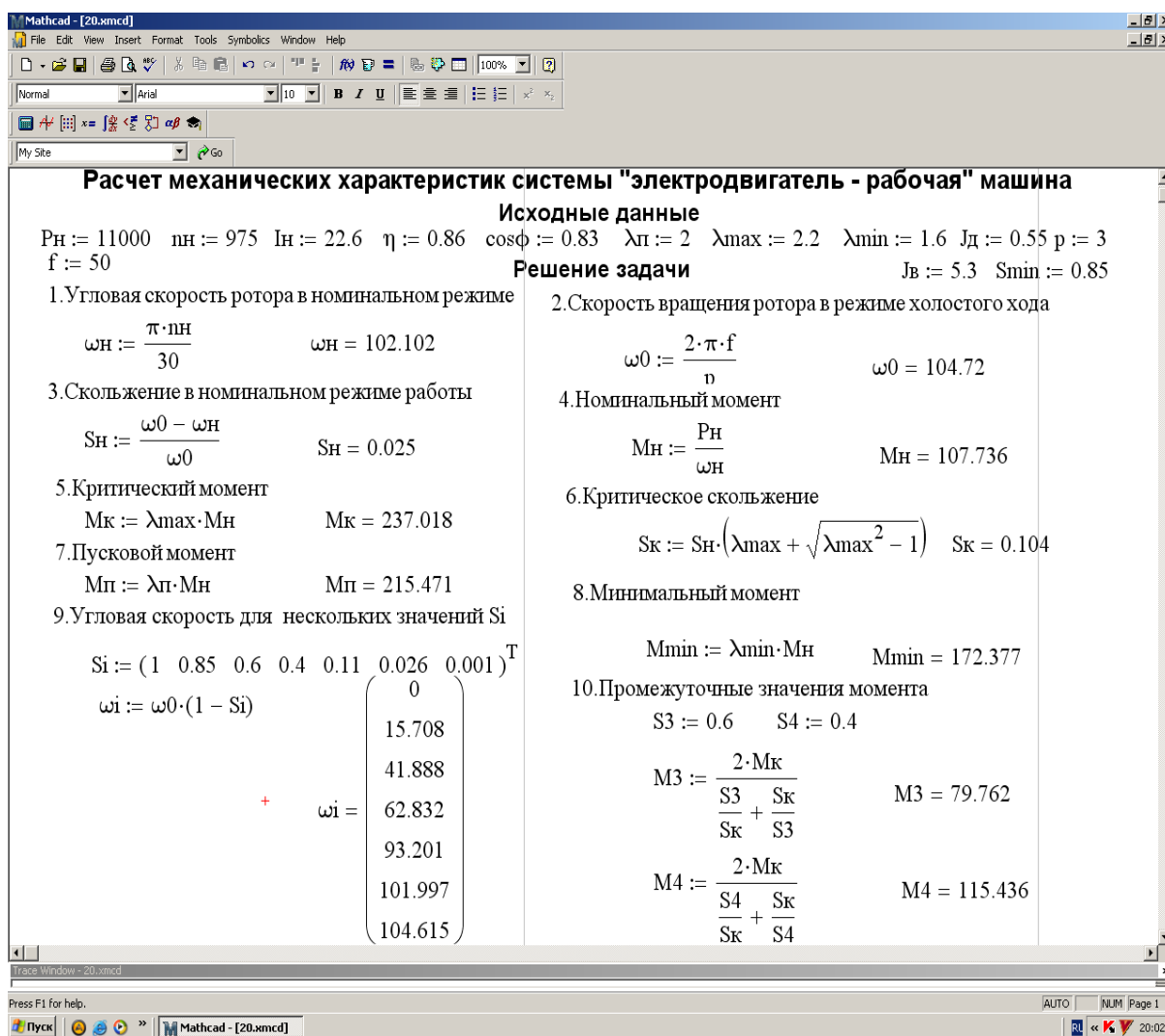
Рисунок 7.23 – Расчет механических характеристик электропривода вентилятора
