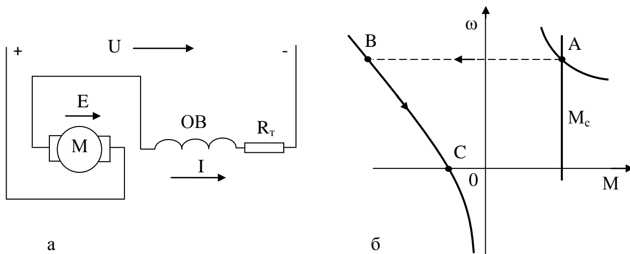
Рисунок 2.26 – Схема подключения (а) и механические характеристики (б) ДПТ ПВ при торможении противовключением
