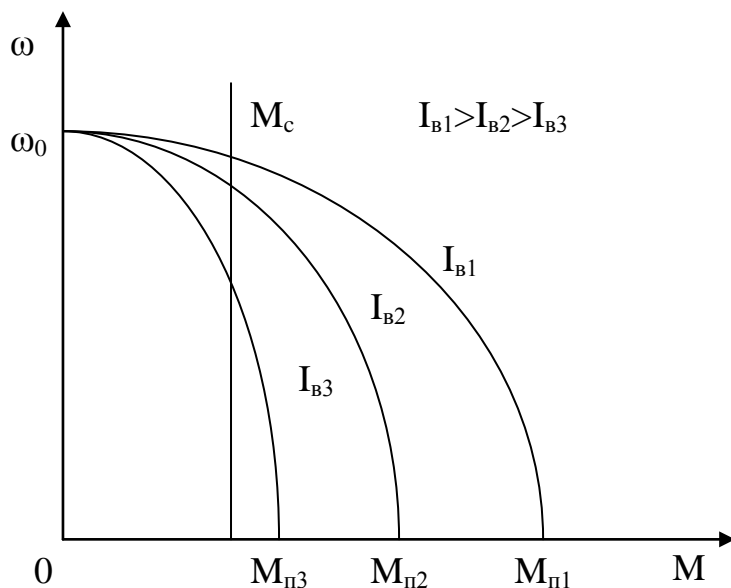
Рисунок 3.18 – Механические характеристики электромагнитной муфты
