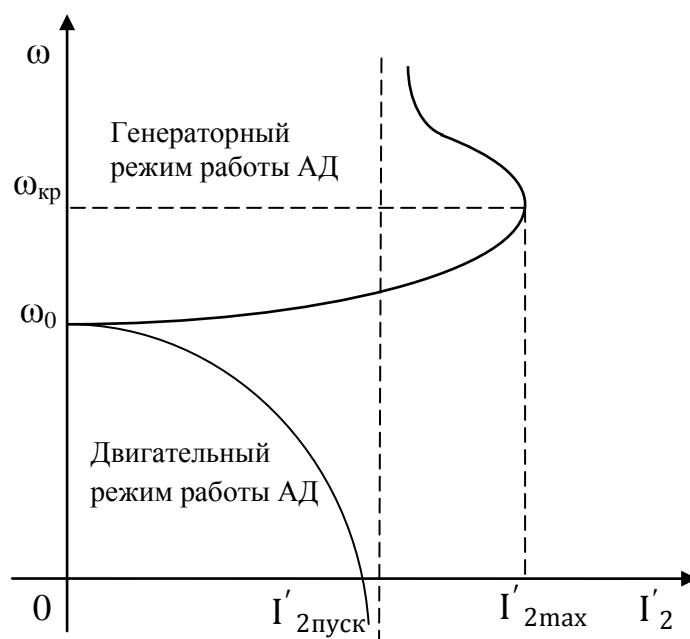
Рисунок 3.4 – Электромеханические характеристики АД в двигательном и генераторном режимах работы
