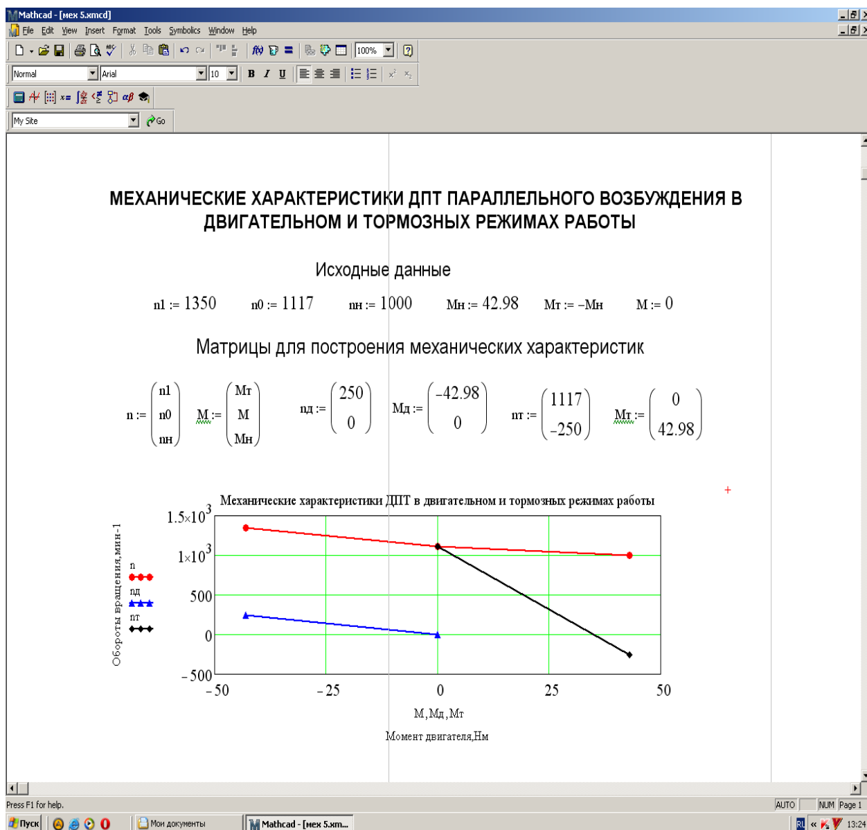
Рисунок 7.5 – Механические характеристики ДПТ с параллельным возбуждением в двигательном и тормозных режимах работы
