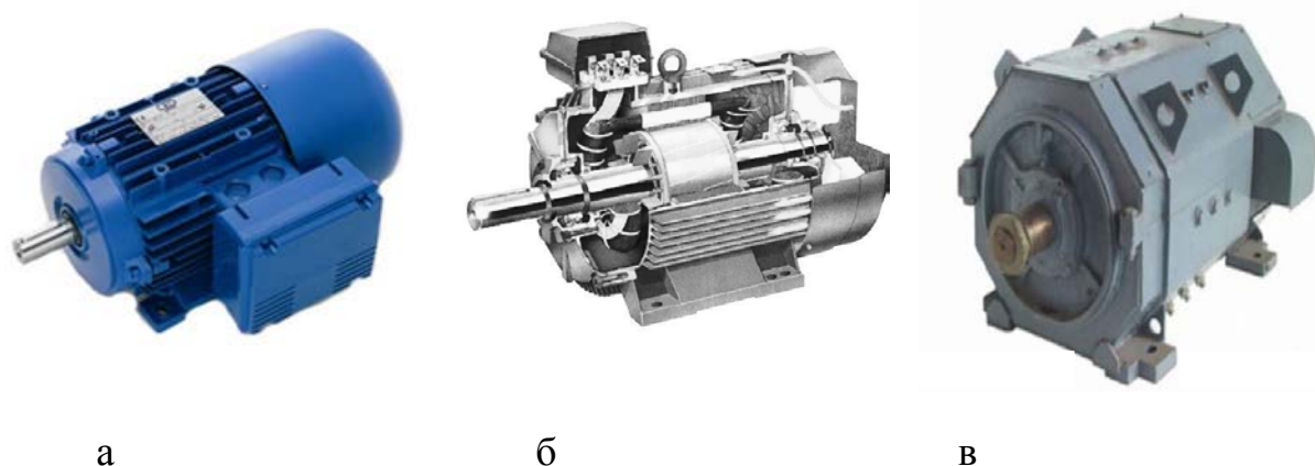
Рисунок 1.7 – Внешний вид электродвигателей: а – асинхронный двигатель с короткозамкнутым ротором; б – электродвигатель с фазным ротором; в - машина постоянного тока
