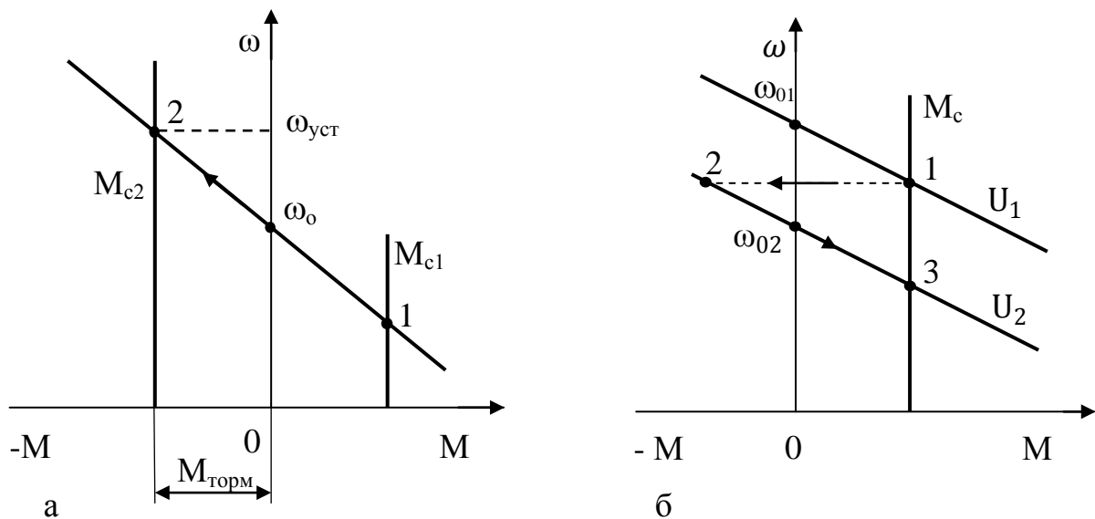
Рисунок 2.18 – Механические характеристики ДПТ НВ в генераторном режиме: а – переход в рекуперативный режим за счет ускорения исполнительного механизма; б - отдача энергии в сеть в результате снижения напряжения
