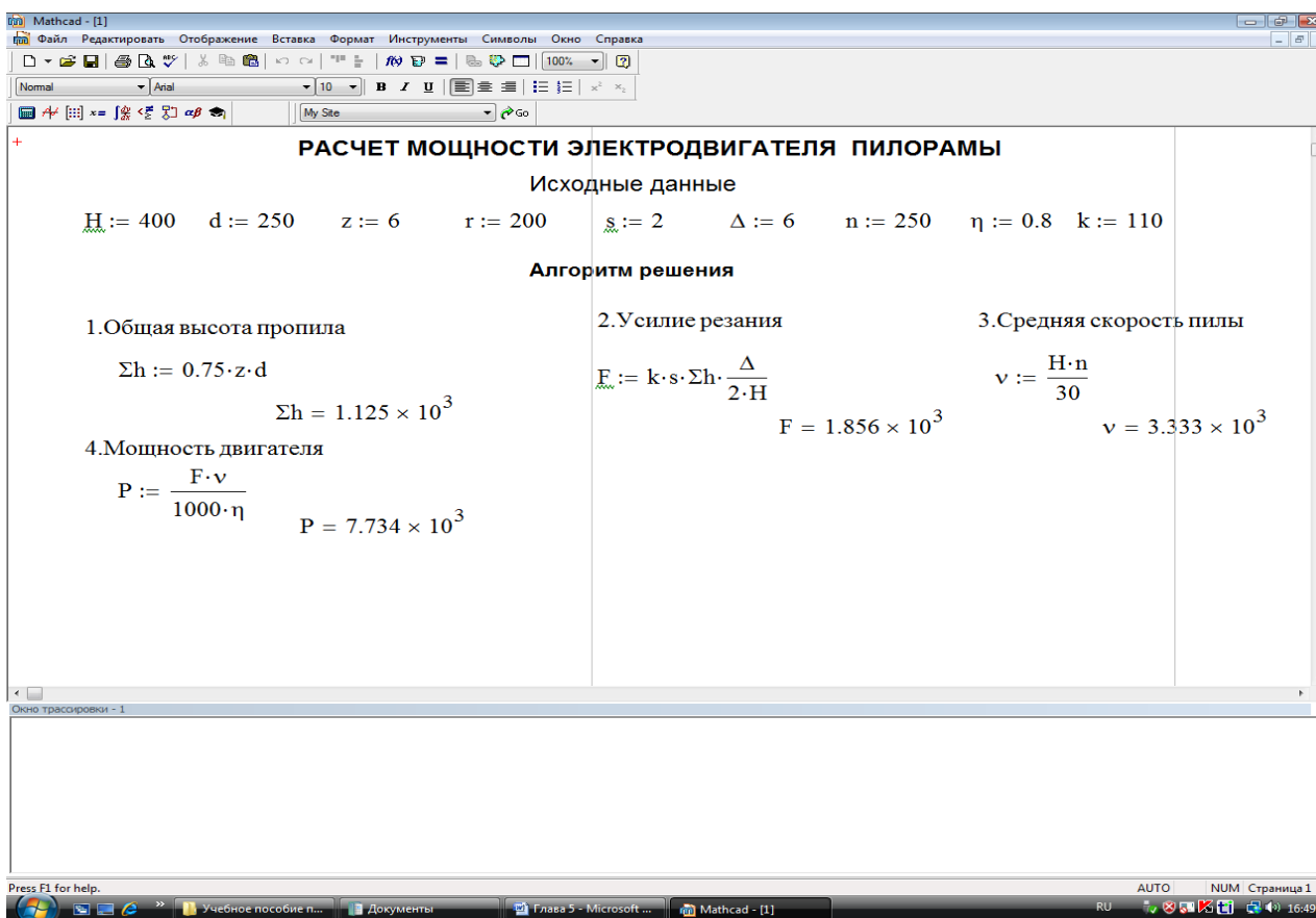
Рисунок 7.22 – Расчет мощности двигателя электропривода пилорамы
