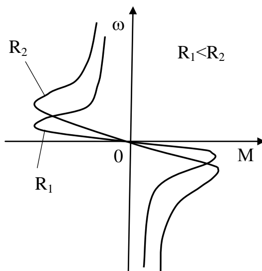
Рисунок 3.23 – Механические характеристики асинхронного двигателя в режиме динамического торможения
