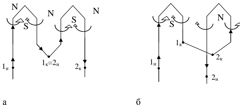
Рисунок 3.13 – Схемы соединения секций одной фазы статорной обмотки АД: а - последовательность соединения начал и концов при p=2 ; б - последовательность соединения начал и концов когда p=1
