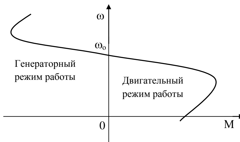
Рисунок 3.19 – Механические характеристики АД в двигательном и генераторном режимах работы
