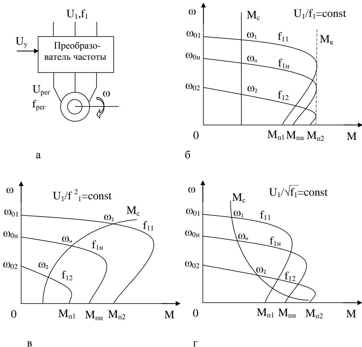
Рисунок 3.12 – Механические характеристики асинхронного электродвигателя при частотном регулировании скорости: а – схема подключения; б – характеристики для нагрузки с постоянным статическим моментом сопротивления; в – характеристики для нагрузки вентиляторного характера; г – характеристики при статическом моменте нагрузки обратно пропорциональном угловой скорости вращения
