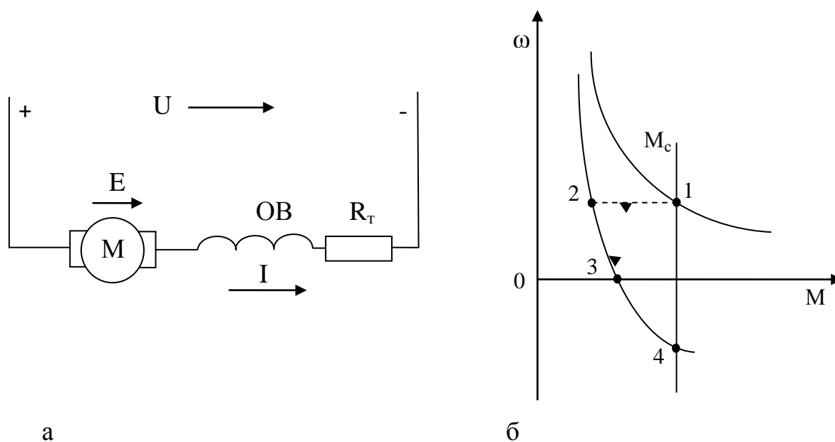
Рисунок 2.27 – Схема подключения (а) и механические характеристики (б) ДПТ ПВ при спуске груза в режиме торможения противовключением
