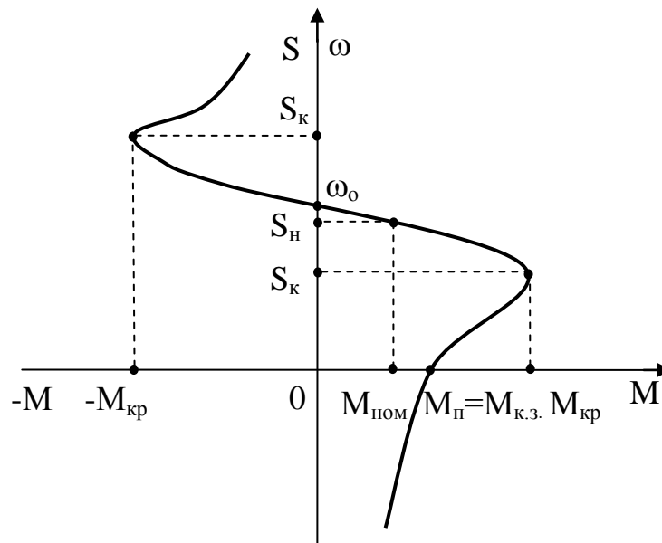
Рисунок 3.5 – Механическая характеристика АД в двигательном и генераторном режимах работы, а также в режиме противовключения
