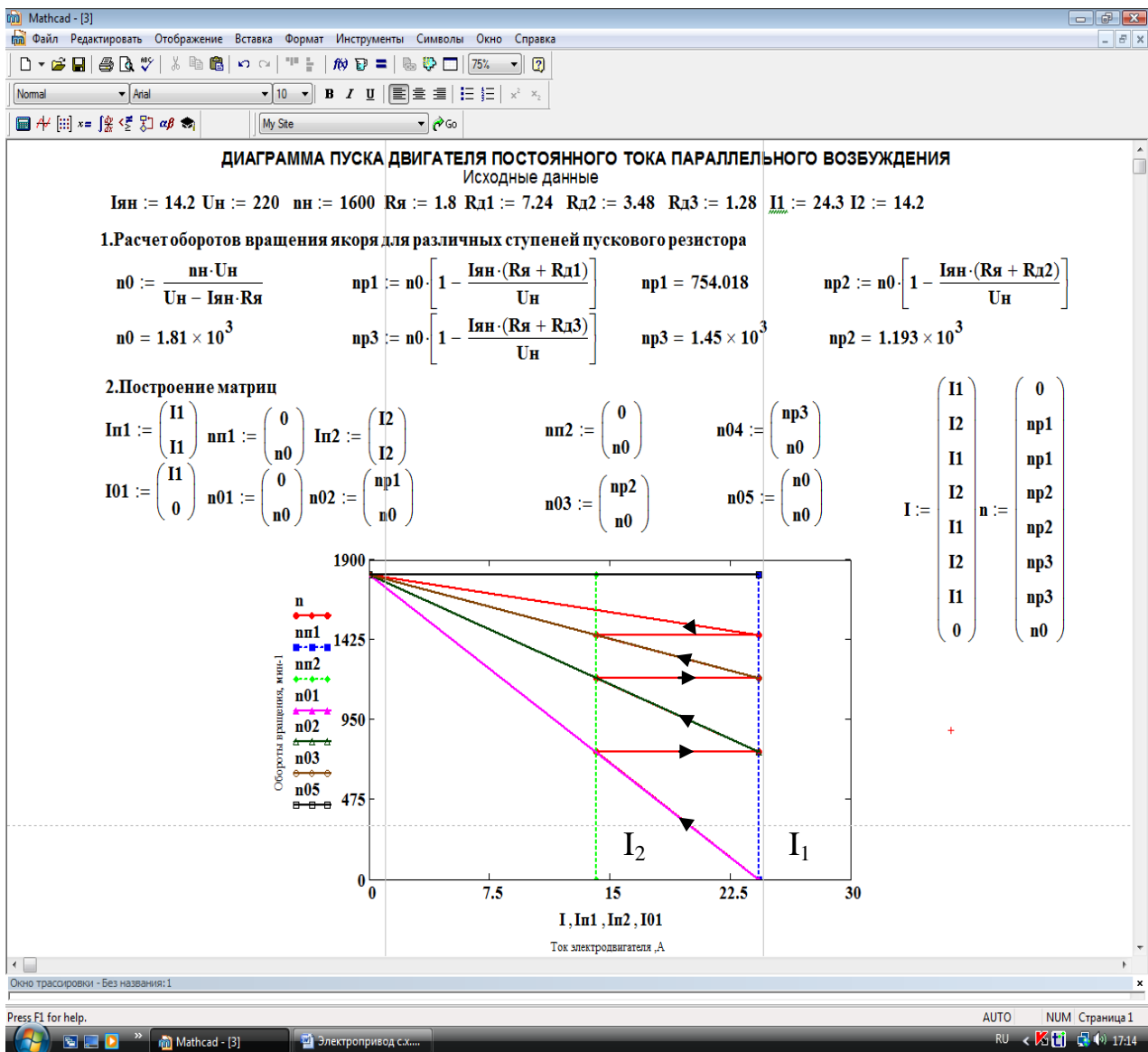
Рисунок 7.7 – Диаграмма пуска двигателя постоянного тока параллельного возбуждения
