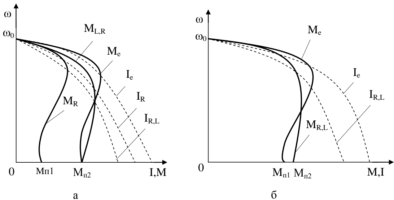
Рисунок 3.11 - Электромеханические и механические характеристики АД с фазным ротором при последовательном (а), параллельном (б) соединении добавочных активных и индуктивных сопротивлений в сравнении с естественной характеристикой
