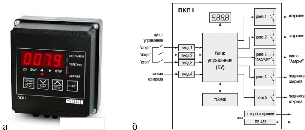
Рисунок 1.4 – Устройство управления электроприводом задвижки: а – передняя панель прибора, б – функциональная схема микропроцессорного устройства управления ПКП1
