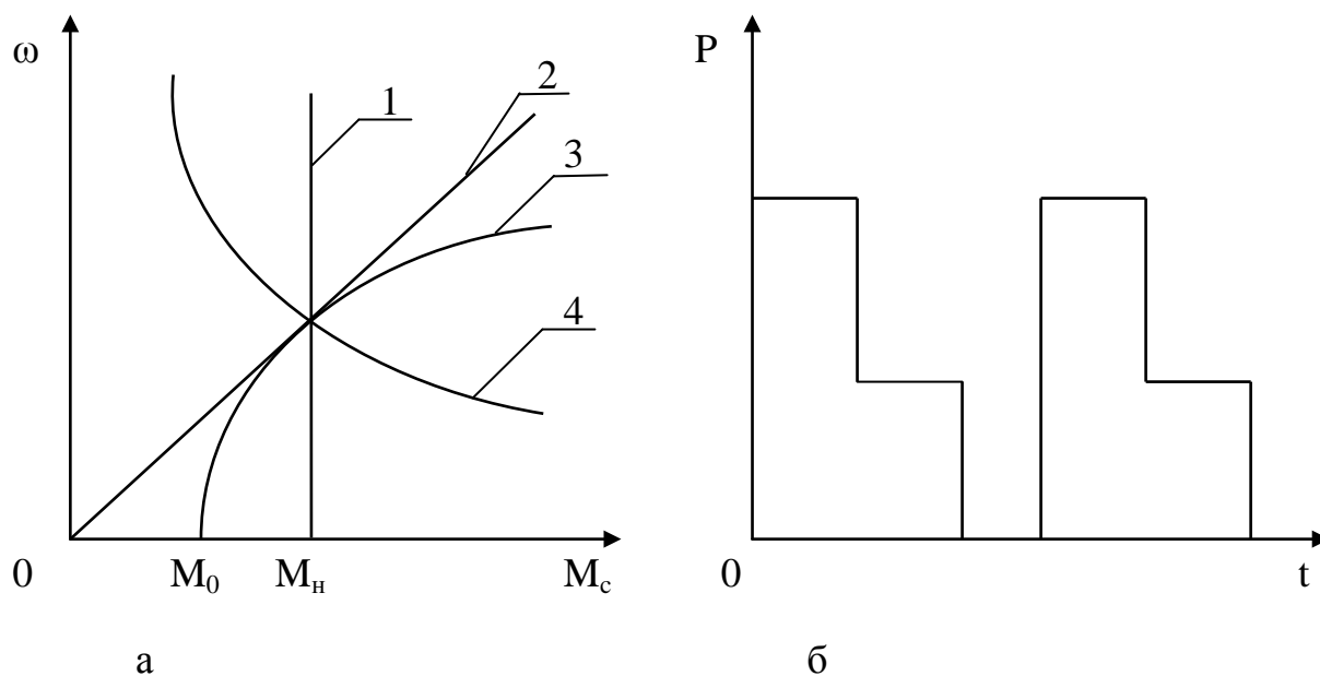
Рисунок 6.1 – Приводные характеристики рабочих машин:
