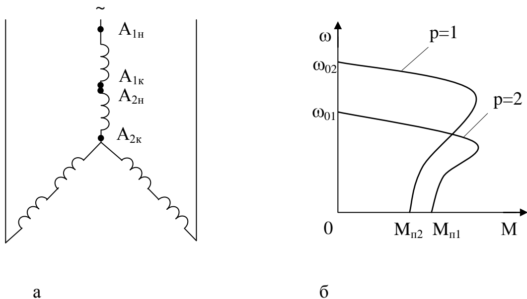
Рисунок 3.15 – Схема соединений секций фаз АД и механические характеристики: а – подключение шести статорных полуобмоток по схеме звезда, б – механические характеристики двухскоростного асинхронного электродвигателя
