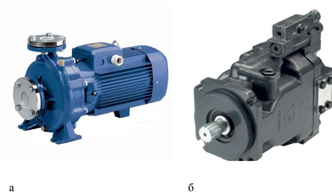
Рисунок 6.2 – Насосные установки: а – центробежный насос; б – аксиально-поршневой насос
