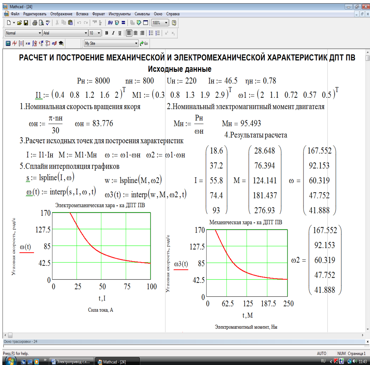
Рисунок 7.10 – Алгоритм расчета, электромеханическая и механическая характеристики ДПТ ПВ
