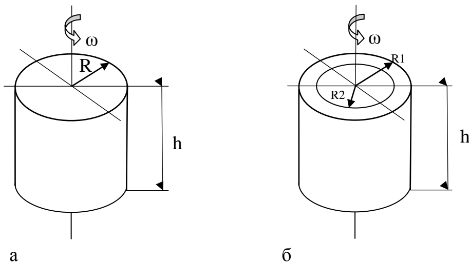
Рисунок 4.3 – Геометрические фигуры, наиболее часто используемые в виде описания маховых масс электропривода: а – цилиндр; б – полый цилиндр
