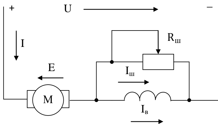
Рисунок 2.11 – Схема подключения ДПТ ПВ с шунтирующим обмотку возбуждения резистором
