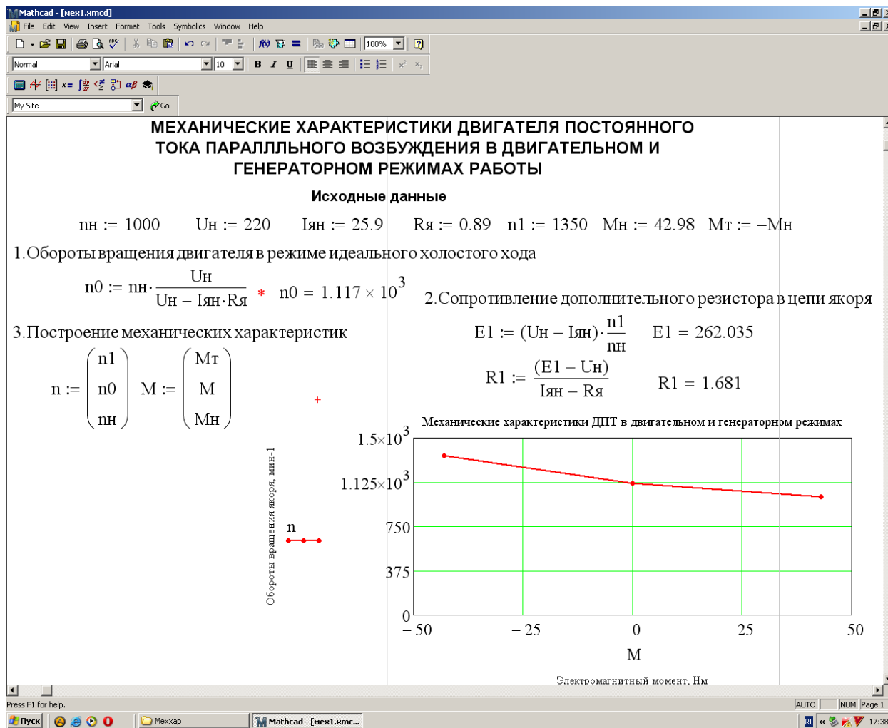
Рисунок 7.2 – Механические характеристики ДПТ параллельного возбуждения в двигательном и генераторном режимах работы
