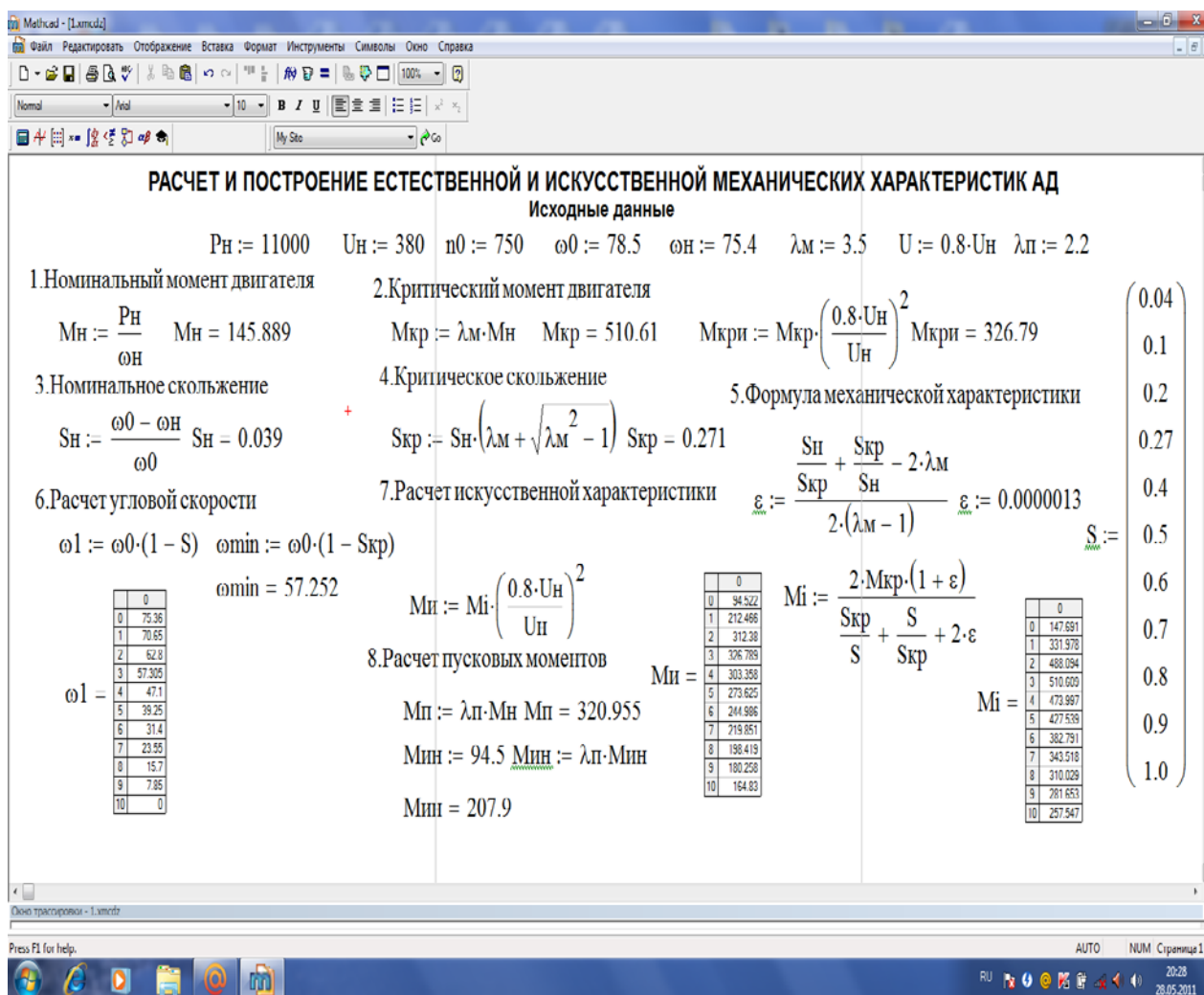
Рисунок 7.14 – Расчет естественной и искусственной механических характеристик АД
