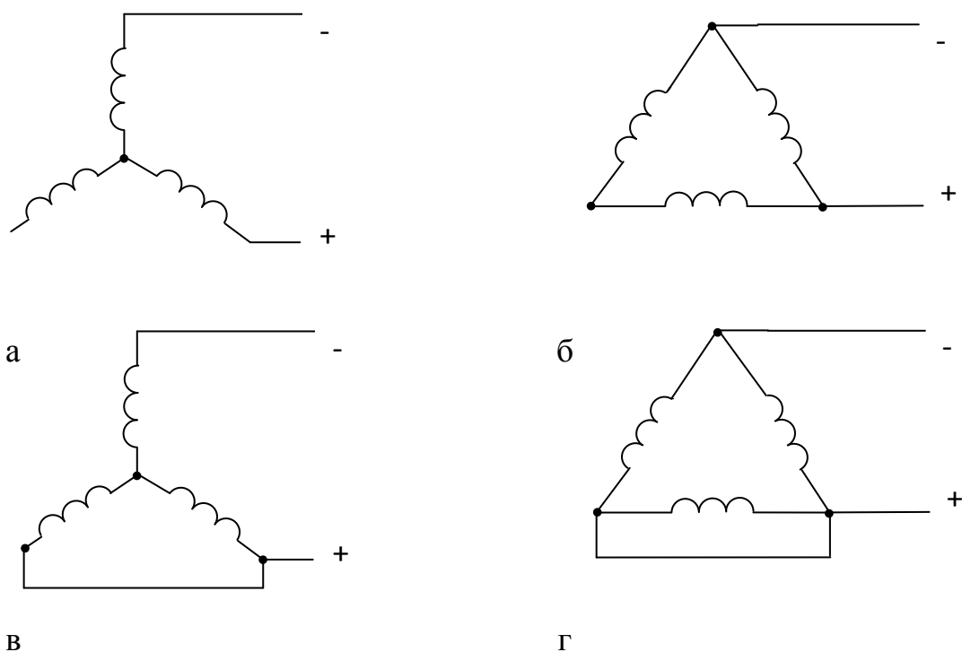
Рисунок 3.22 – Варианты схем питания статора асинхронного двигателя постоянным током при электродинамическом торможении
