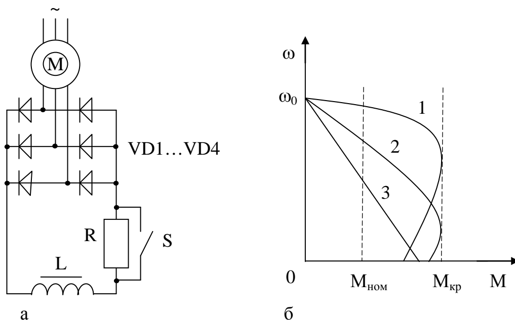
Рисунок 3.16 – Схема подключения формирователя импульсного напряжения (а) и механические характеристики (б) АД с фазным ротором
