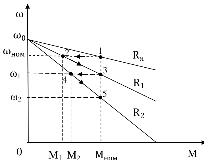
Рисунок 2.5 - Регулирование угловой частоты вращения изменением сопротивления в цепи якоря: R_2 > R_1 > R_я
