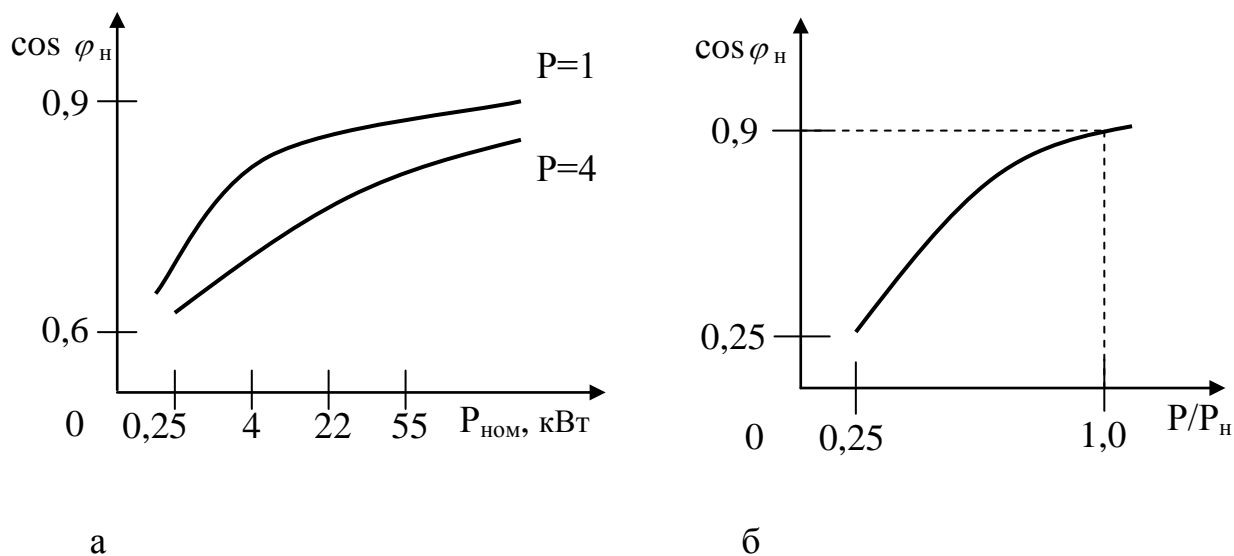
Рисунок 5.2 – Изменение \cos \varphi электродвигателей: а – график \cos \varphi в функции мощности; б – зависимость \cos \varphi от величины загрузки электродвигателя
