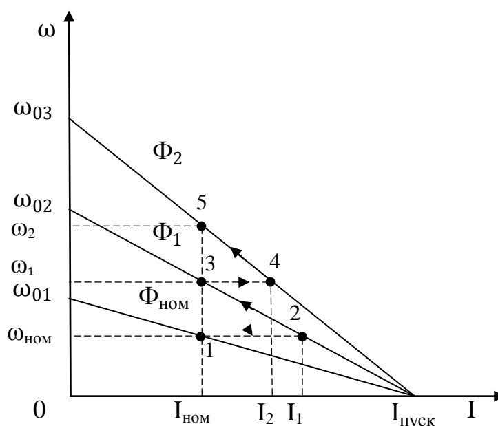
Рисунок 2.6 – Электромеханические характеристики, построенные в результате изменения магнитного потока
