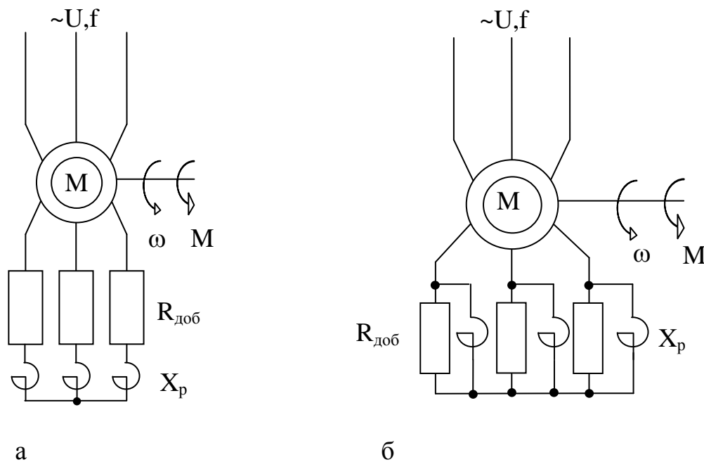
Рисунок 3.10 – Схемы запуска асинхронного двигателя при наличии дополнительных индуктивного и активного сопротивлений в цепи якоря: а – последовательное соединение; б – параллельное подключение
