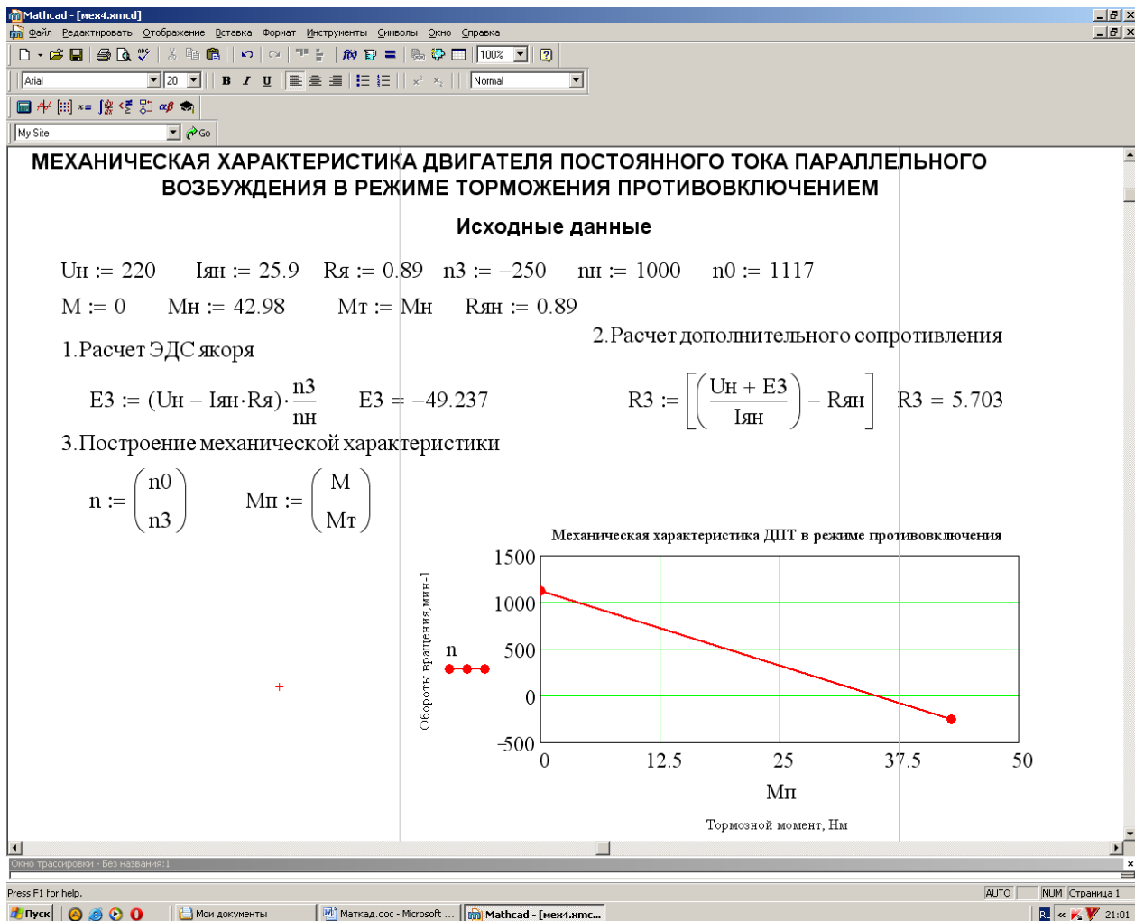
Рисунок 7.4 – Механическая характеристика двигателя постоянного тока в режиме торможения противоблокировкой
