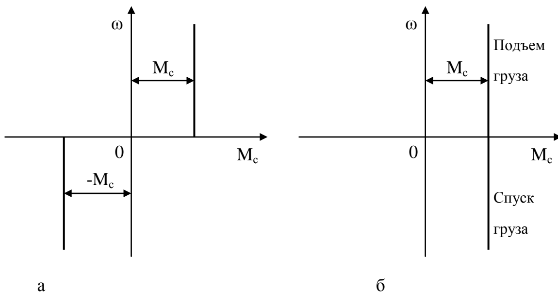
Рисунок 4.1 – Графики статических моментов сопротивления:
