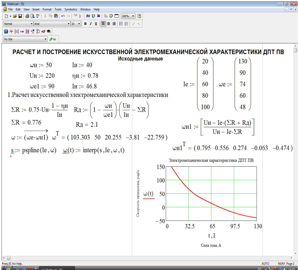
Рисунок 7.11 – Электромеханическая характеристика ДПТ ПВ
