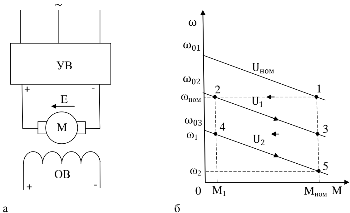
Рисунок 2.8 - Схема управления ДПТ НВ (а), механические характеристики (б), полученные в результате изменения напряжения, U_{\text{НОМ}} > U_1 > U_2
