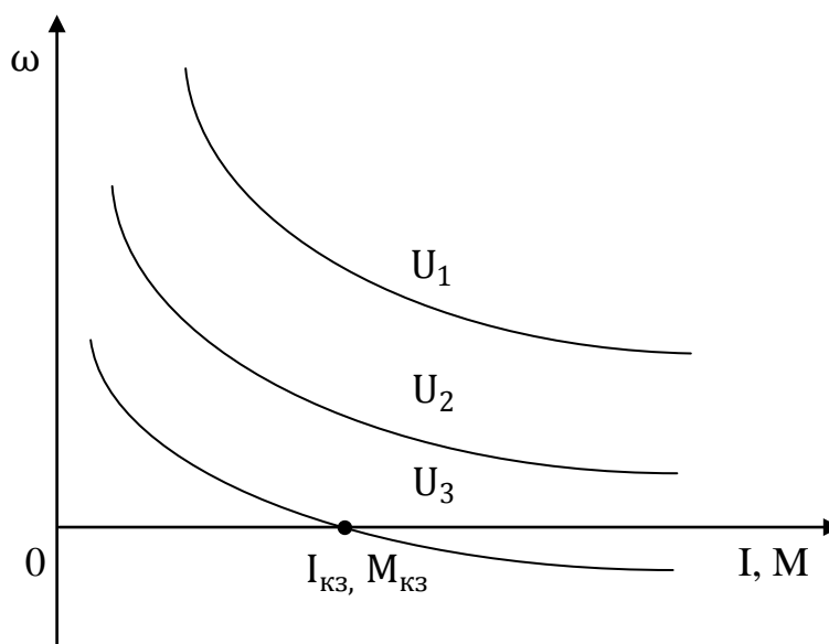
Рисунок 2.10 – Механические и электромеханические характеристики ДПТ ПВ: U_1 – естественная; U_2, U_3 - искусственные характеристики, U_1 > U_2 > U_3
