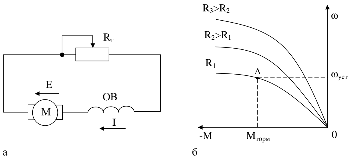
Рисунок 2.22 – Схема подключения (а) и механические характеристики (б) ДПТ ПВ в режиме динамического торможения с самовозбуждением
