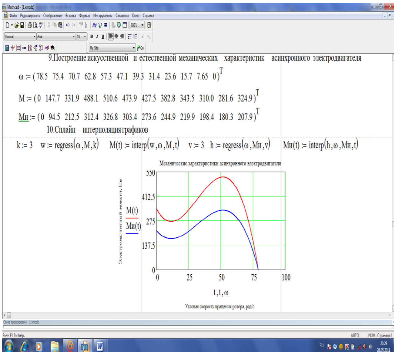
Рисунок 7.15 – Построение естественной и искусственной механических характеристик асинхронного электродвигателя
