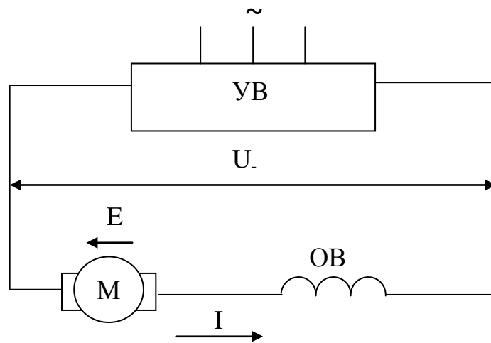
Рисунок 2.13 – Схема подключения ДПТ ПВ к управляемому выпрямителю
