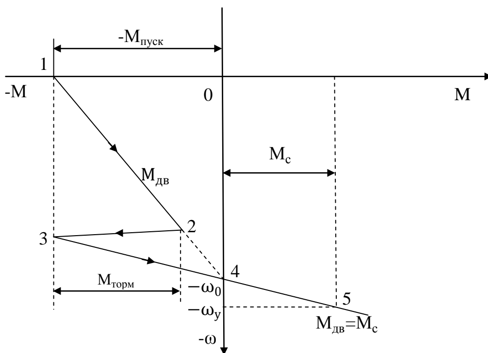
Рисунок 2.19 – Механические характеристики ДПТ НВ при спуске груза
