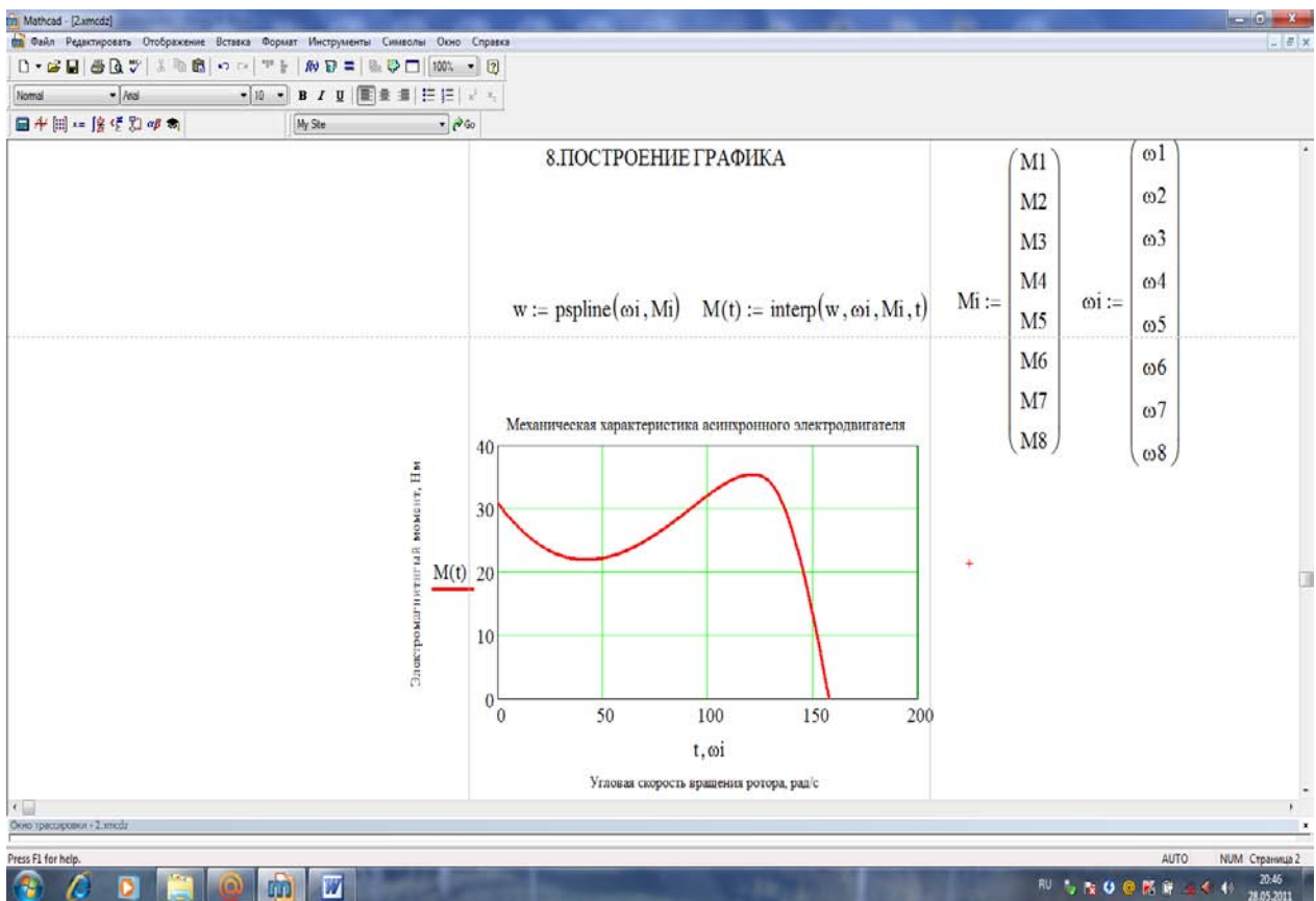
Рисунок 7.13 – Механическая характеристика асинхронного двигателя
