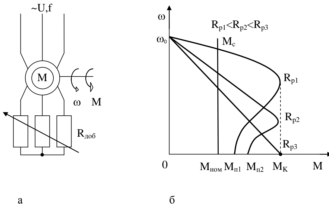
Рисунок 3.9 – Упрощенная схема подключения резисторов (а) асинхронного двигателя с фазным ротором и механические (б) характеристики
