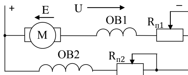
Рисунок 2.16 – Схема подключения двигателя постоянного тока смешанного возбуждения
