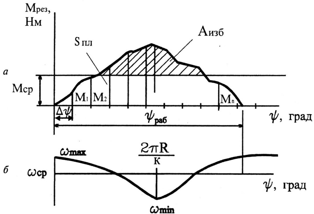
Рисунок 6.12 - Диаграмма моментов резания и угловой скорости рабочего барабана
