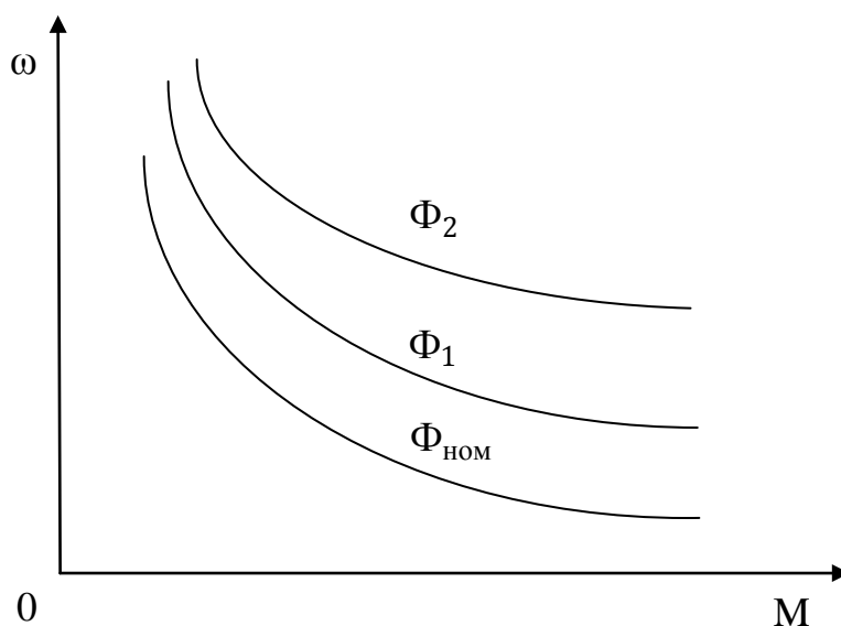
Рисунок 2.12 – Естественная и искусственные механические характеристики ДПТ ПВ с шунтированием обмотки возбуждения,
