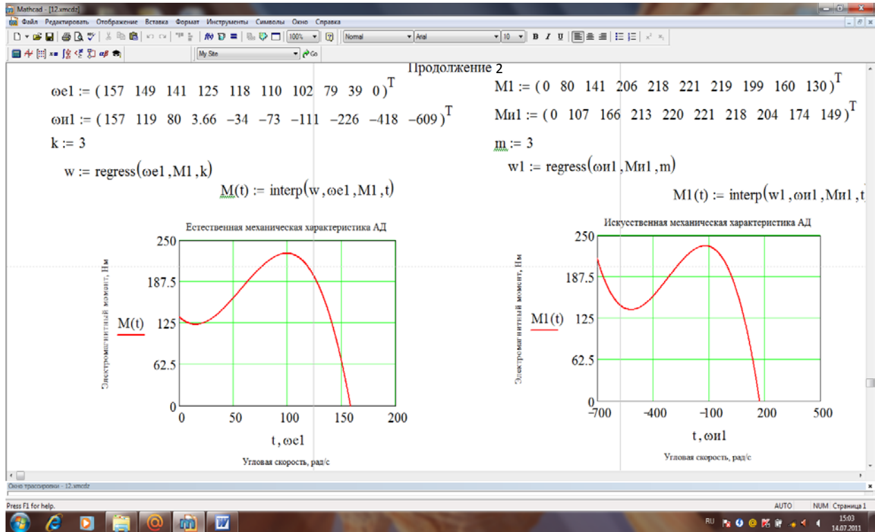
Рисунок 7.18 – Построение механических характеристик АД
