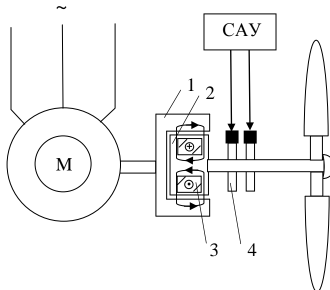
Рисунок 3.17 – Асинхронный короткозамкнутый двигатель с электромагнитной муфтой скольжения
