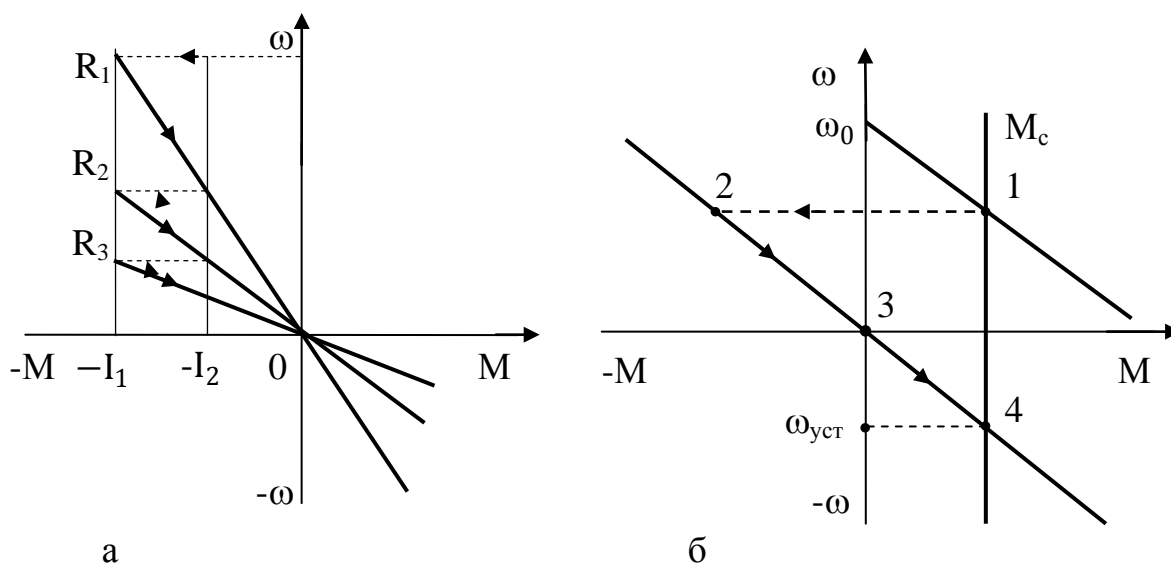
Рисунок 2.21 – Механические характеристики ДПТ НВ в режиме динамического торможения: а – характеристики, полученные при замыкании обмотки якоря на многоступенчатое тормозное сопротивление; б – характеристики, построенные в результате спуска груза
