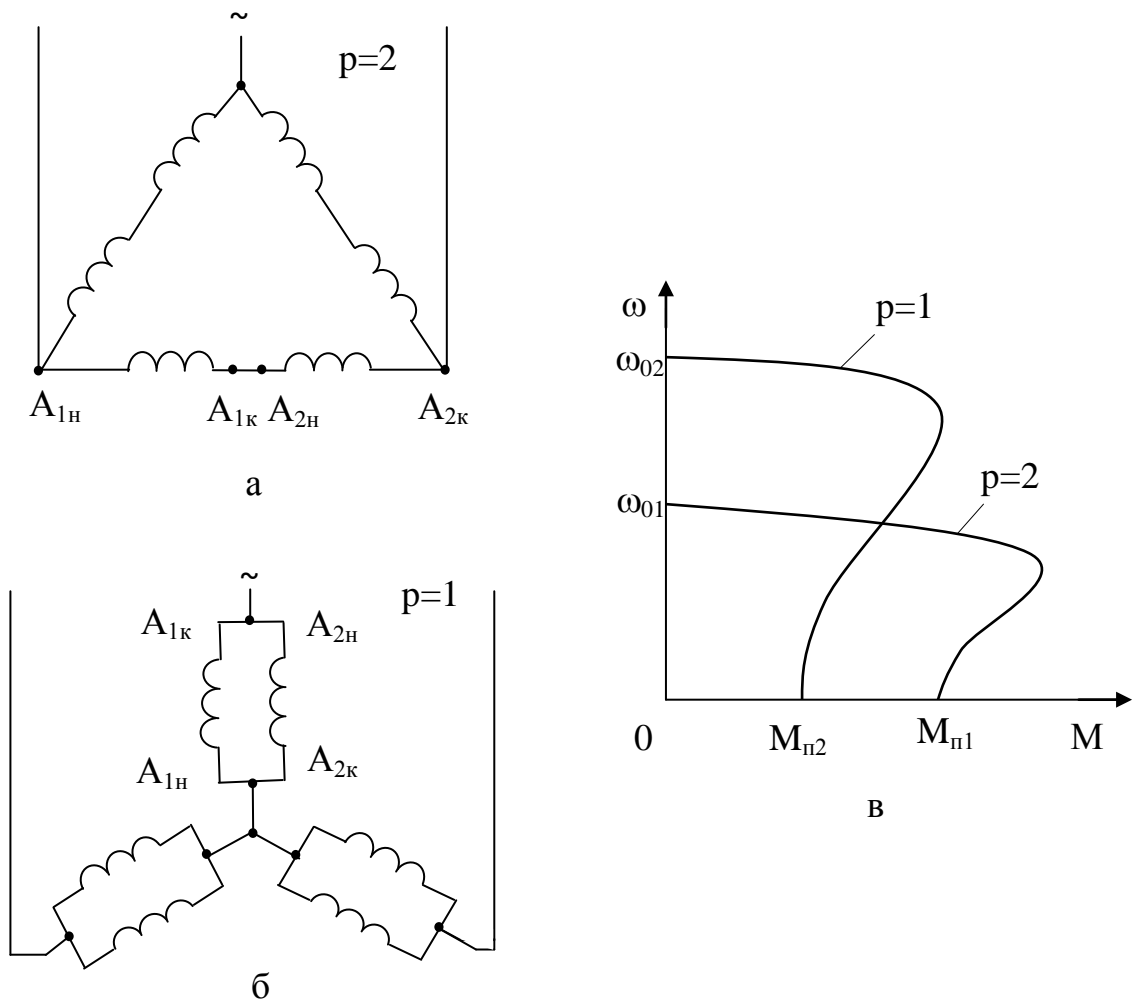
Рисунок 3.14 – Схемы соединения обмоток и характеристики асинхронного электродвигателя с короткозамкнутым ротором: а – соединение секций статора по схеме треугольник; б – соединение катушек по схеме двойная звезда; в – механические характеристики двухскоростного двигателя, имеющего разные значения числа полюсов
