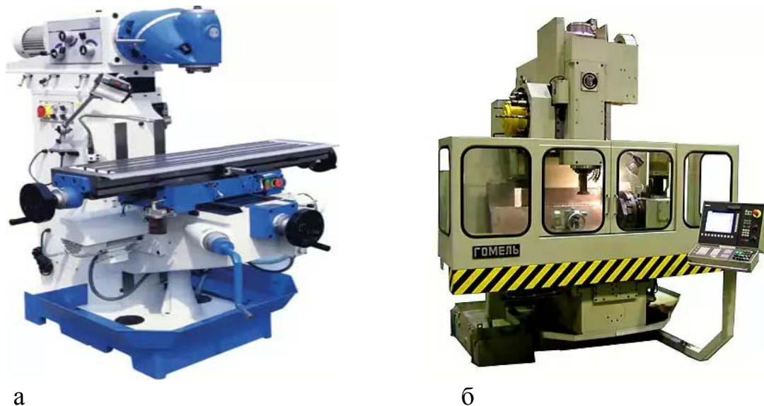
Рисунок 6.16 – Фрезерно-обрабатывающие станки: а – фрезерный станок с асинхронным приводом; б – автоматизированный фрезерный центр с ЧПУ
