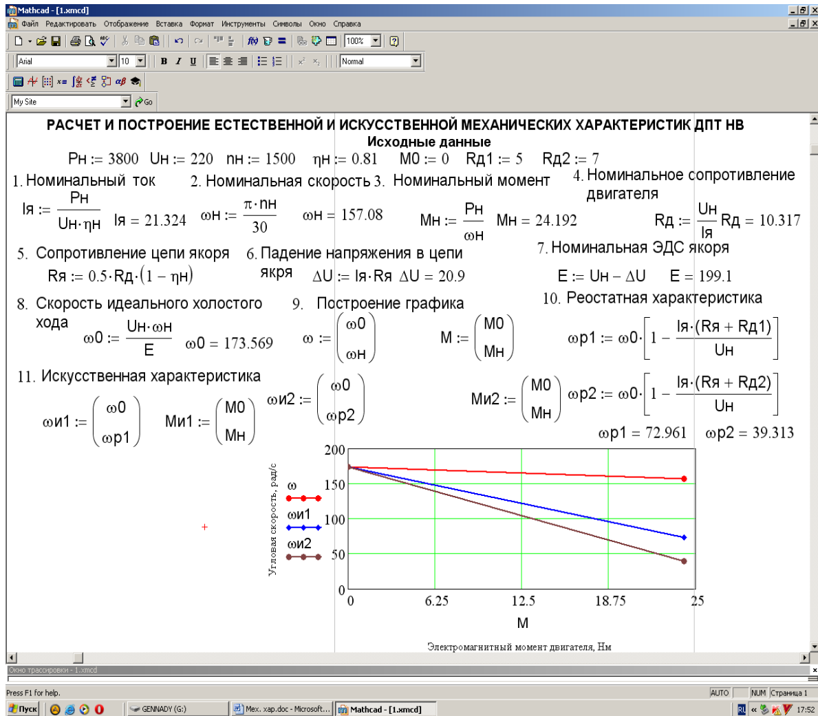
Рисунок 7.8 – Расчет и построение естественной и искусственных механических характеристик ДПТ НВ
