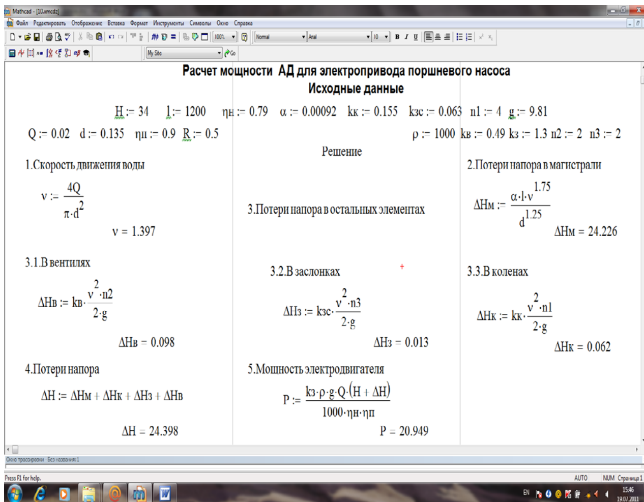
Рисунок 7.20 – Расчет мощности электродвигателя поршневого насоса
