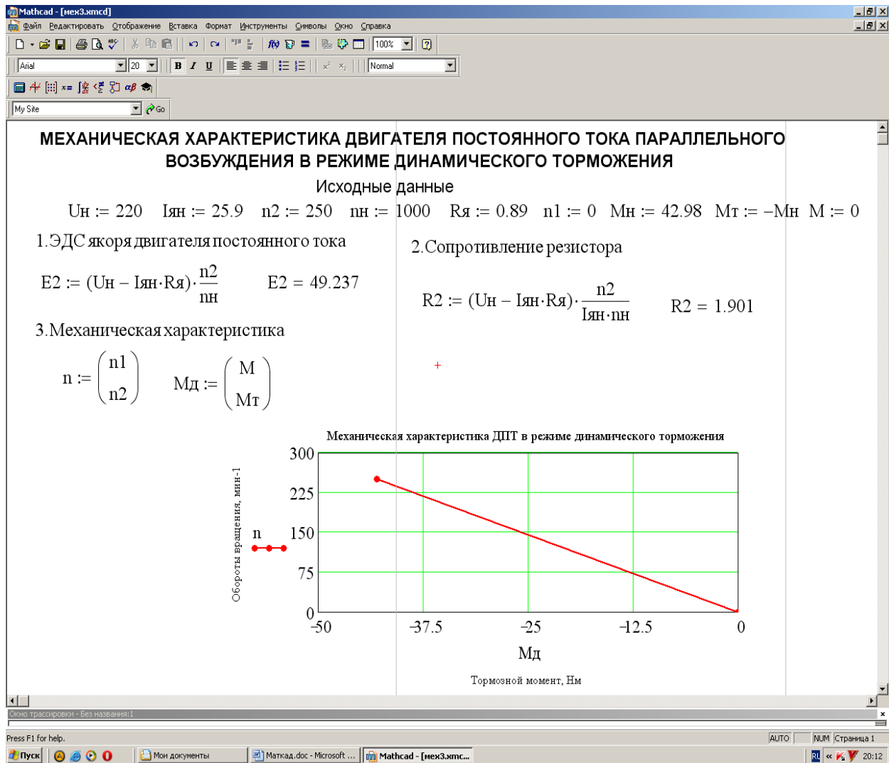
Рисунок 7.3 – Механическая характеристика ДПТ в режиме динамического торможения
