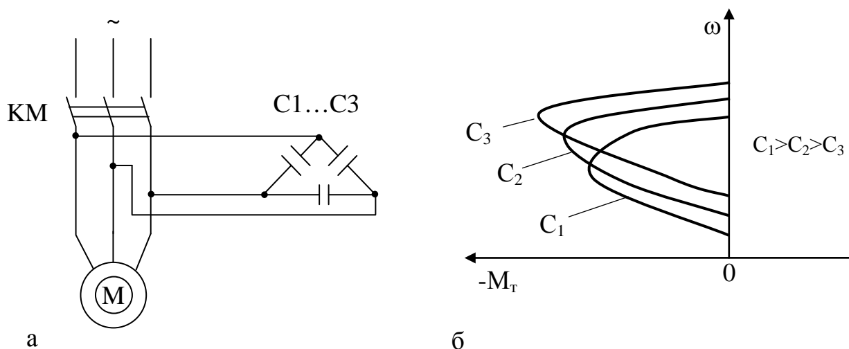
Рисунок 3.24 – Схема подключения (а) и механические характеристики (б) АД в режиме динамического торможения с самовозбуждением
