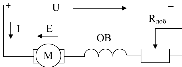
Рисунок 2.9 – Схема подключения двигателя постоянного тока с последовательной обмоткой возбуждения
