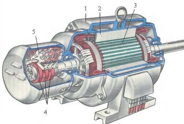
Рисунок 3.2 – Асинхронный электродвигатель с фазной обмоткой ротора:
