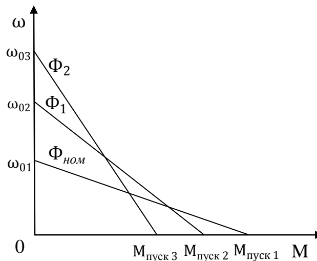
Рисунок 2.7 - Механические характеристики ДПТ НВ
