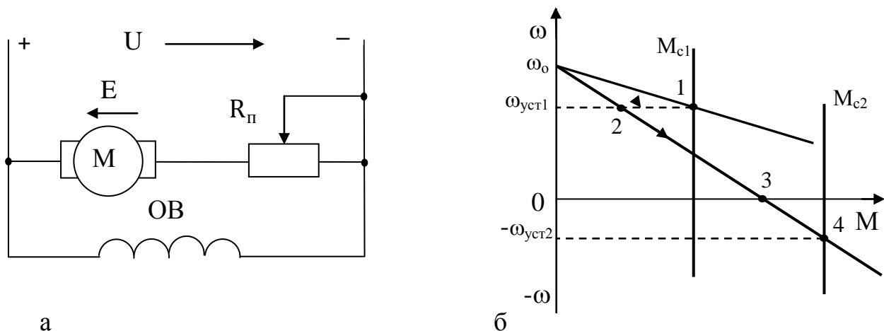
Рисунок 2.23 – Схема включения ДПТ НВ в режиме противовключения (а) и механическая характеристика (б)
