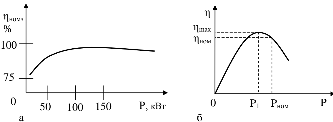
Рисунок 5.1 – Графики КПД электродвигателя: а – КПД в функции мощности; б – зависимость КПД от величины нагрузки на выходном валу двигателя
