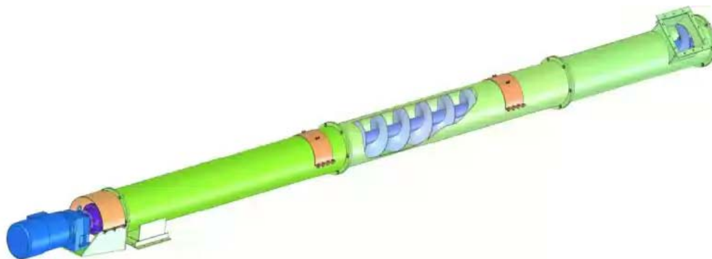
Рисунок 6.6 – Внешний вид шнекового цилиндрического транспортера
