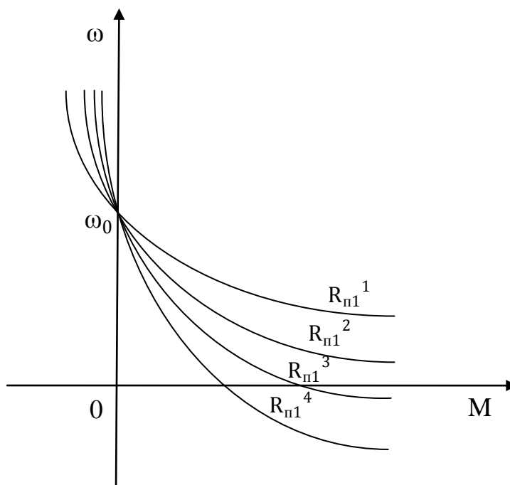
Рисунок 2.17 – Механические характеристики ДПТ СВ,
