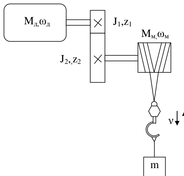
Рисунок 4.2 – Кинематическая схема лебедки с электроприводом
