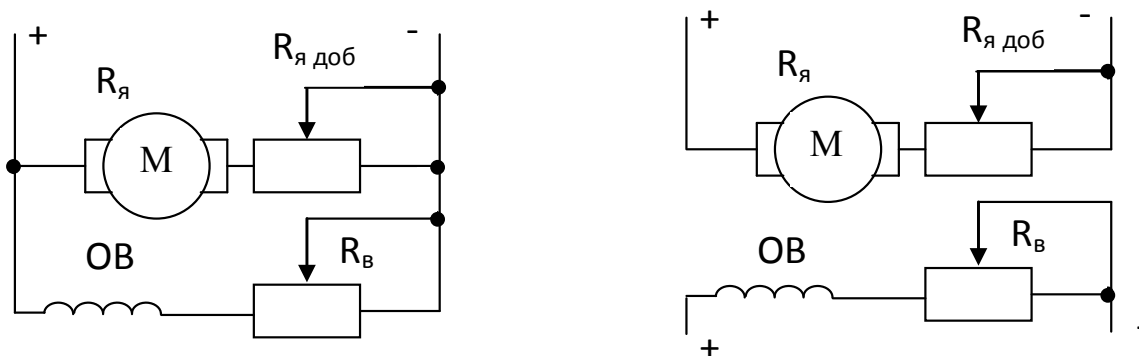
Рисунок 2.3 - Схемы подключения ДПТ с параллельной и независимой обмоткой возбуждения
