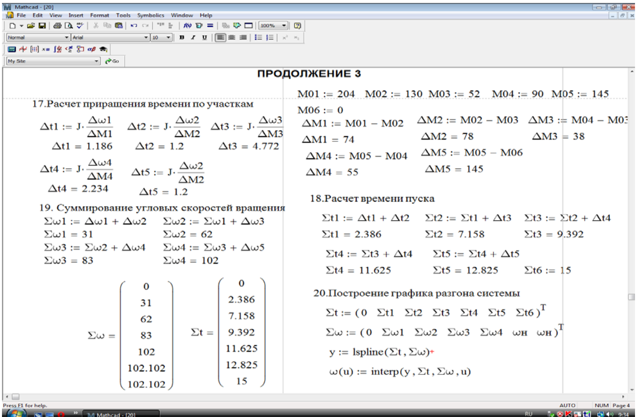
Рисунок 7.26 – Расчет приращения времени разгона по участкам
