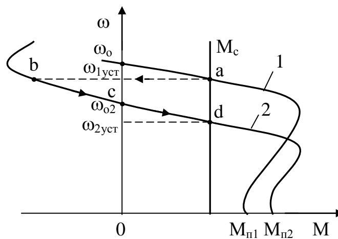
Рисунок 3.20 – Механические характеристики асинхронной машины в режиме генераторного торможения
