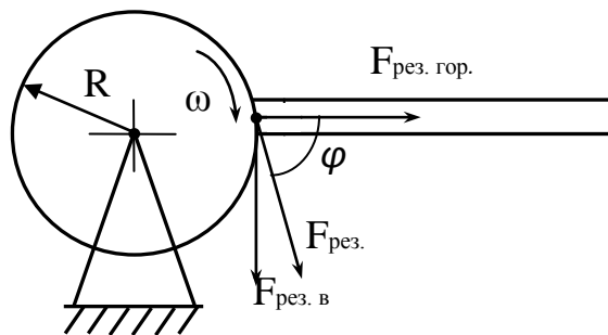
Рисунок 6.18 – Схема подачи и направления усилий в момент распиловки бревен
