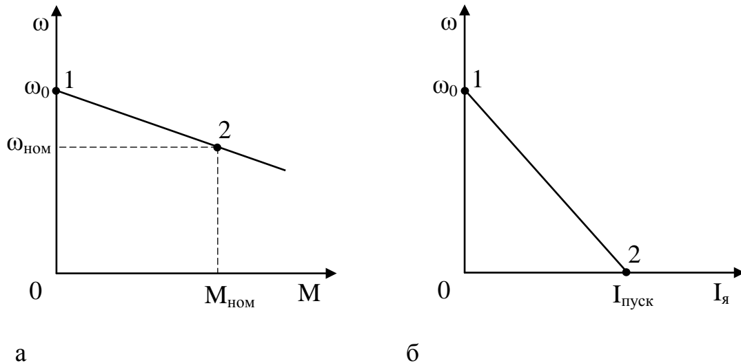
Рисунок 2.4 - Механическая (а) и электромеханическая (б) характеристики ДПТ НВ
