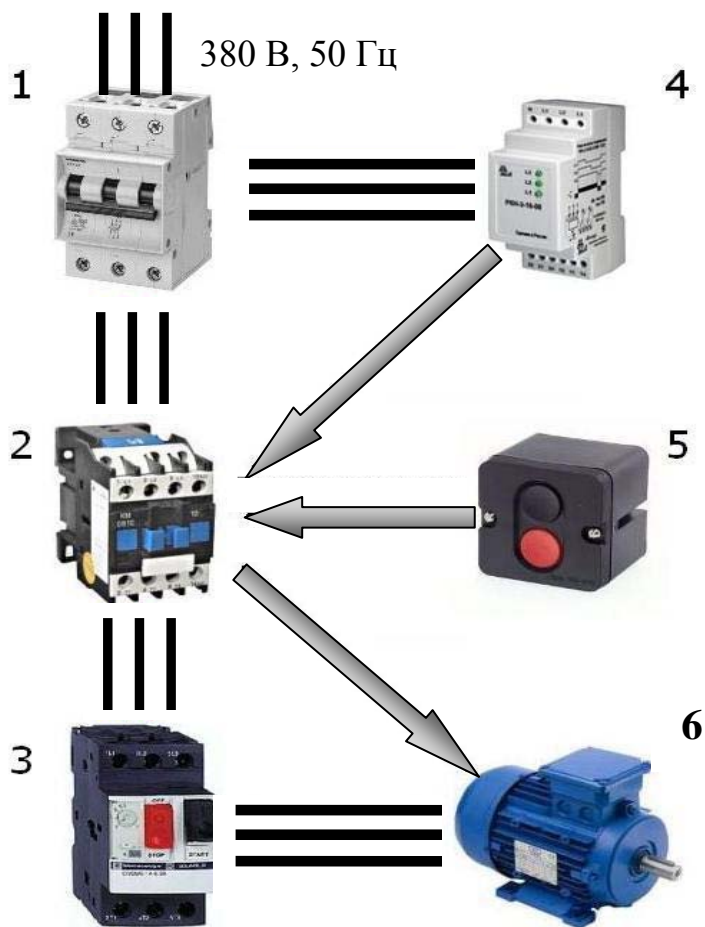
Рисунок 1.2 – Упрощенная схема подключения асинхронного электропривода: 1 - вводной автоматический выключатель; 2 - магнитный пускатель; 3 - тепловое реле; 4 - реле контроля фаз и уровня напряжения; 5 - кнопки управления; 6 - электродвигатель
