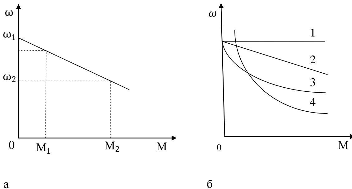
Рисунок 2.2 – Механические характеристики электродвигателей: а – иллюстрация к определению жесткости; б – механические характеристики электродвигателей: 1 – абсолютно жесткая синхронного вентильного двигателя; 2 – жесткая двигателя постоянного тока независимого возбуждения; 3 – мягкая двигателя постоянного тока смешанного возбуждения; 4 – мягкая двигателя постоянного тока последовательного возбуждения;
