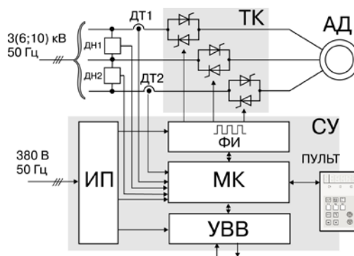
СУ — система управления; МК — микропроцессорный контроллер; ТК — 3-х фазный тиристорный коммутатор; УВВ — устройство ввода-вывода; ИП — источник питания; АД — трехфазный асинхронный двигатель; ФПИ — формирователь управляющих импульсов тиристоров; ДТ1, ДТ2 — датчики тока; ДН1, ДН2 — датчики напряжения.
