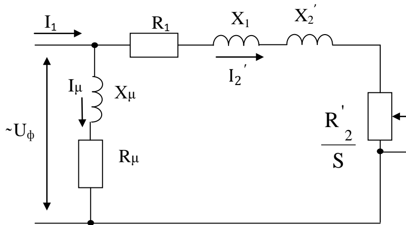
Рисунок 3.3 – Эквивалентная Г – образная схема замещения асинхронного электродвигателя
