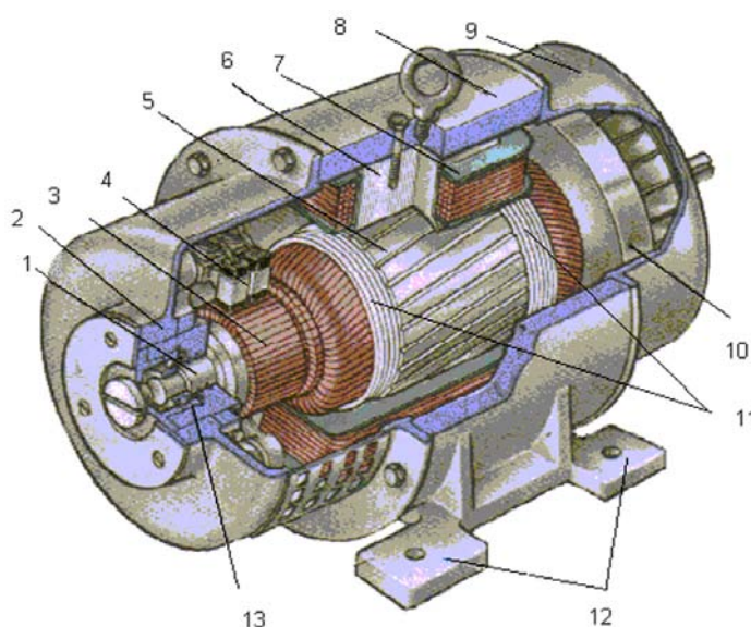
Рисунок 2.1 – Разрез конструкции машины постоянного тока:
