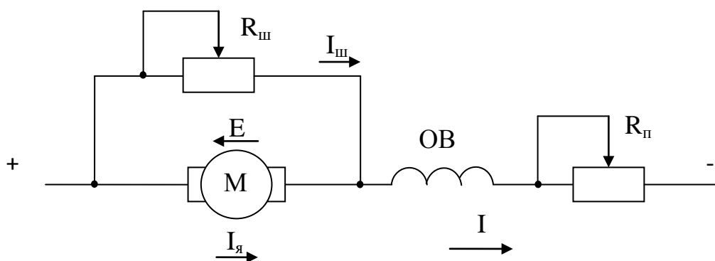
Рисунок 2.14 – Схема подключения ДПТ ПВ с шунтирующей обмотку якоря переменным резистором
