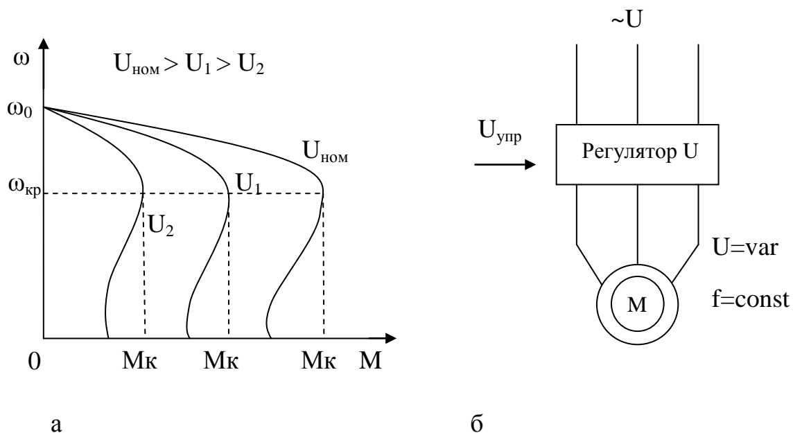
Рисунок 3.6 – Механические характеристики (а) при регулировании напряжения питания АД; упрощенная схема (б) регулятора напряжения
