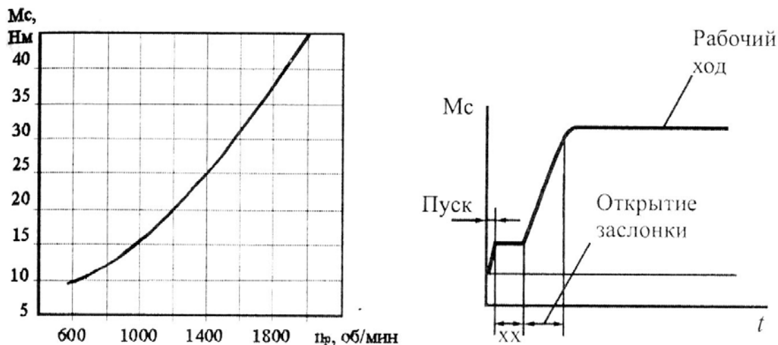
Рисунок 6.11 – Характеристики дробилки: а – механическая; б – нагрузочная
