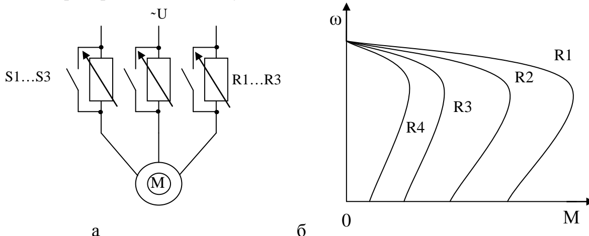
Рисунок 3.8 – Упрощенная схема (а) подключения переменных резисторов в электрические цепи фаз обмотки статора; естественная и искусственные механические характеристики (б) АД: R1 < R2 < R3 < R4
