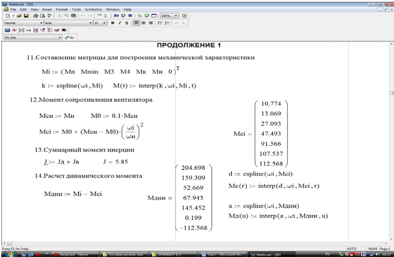
Рисунок 7.24 – Продолжение расчета кривой разгона электропривода вентилятора
