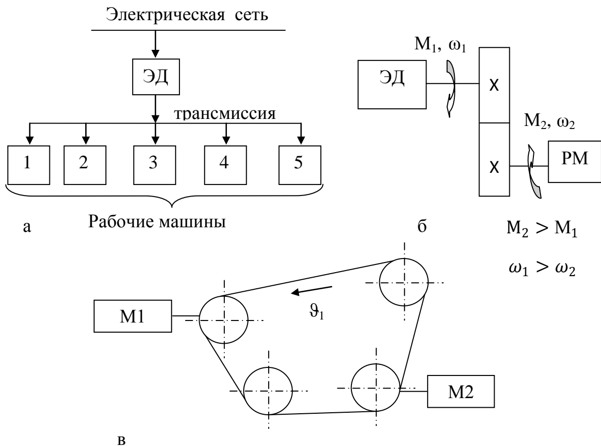
Рисунок 1.10 – Схемы электропривода: а – групповой; б – индивидуальный; в – взаимосвязанный
