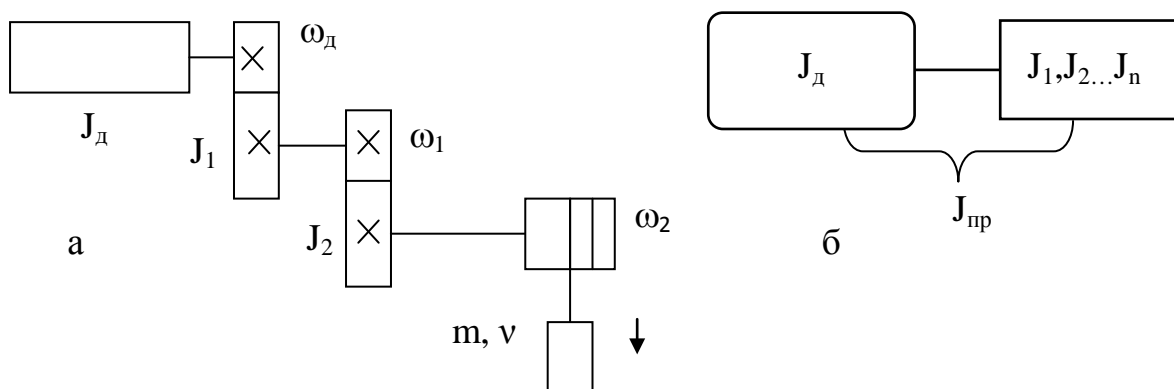
Рисунок 4.4 – Приведение моментов инерции электропривода к валу двигателя: а – кинематическая схема исходной системы; б – система, приведенная к валу электродвигателя
