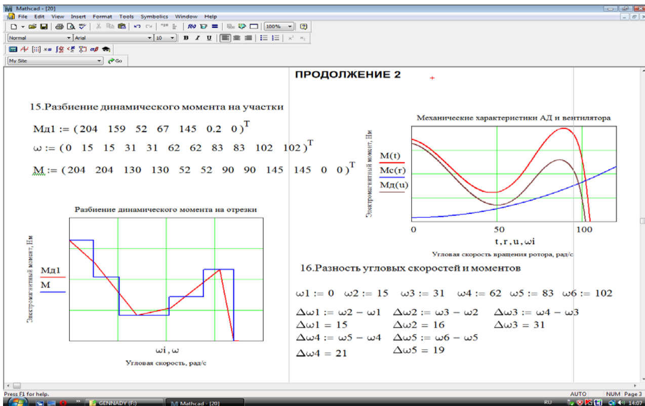
Рисунок 7.25 – Построение механических характеристик электродвигателя и рабочей машины - вентилятора
