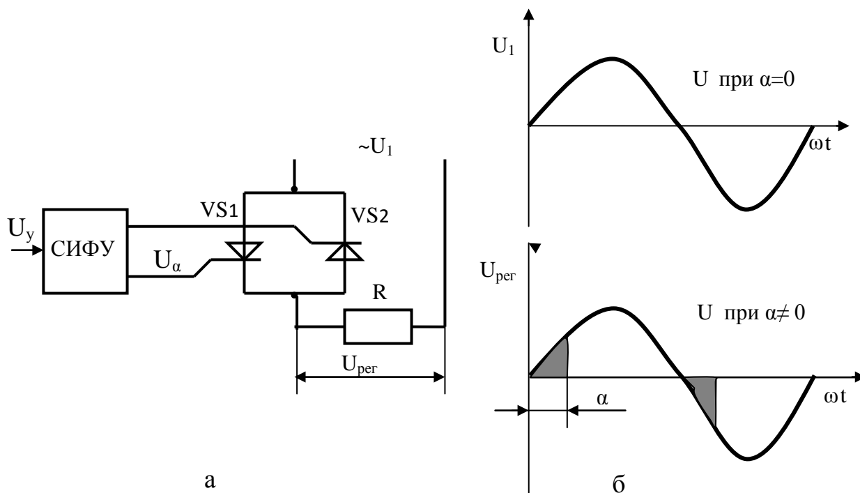
Рисунок 3.7 – Упрощенная схема (а) и синусоиды напряжения (б) однофазного ТРН
