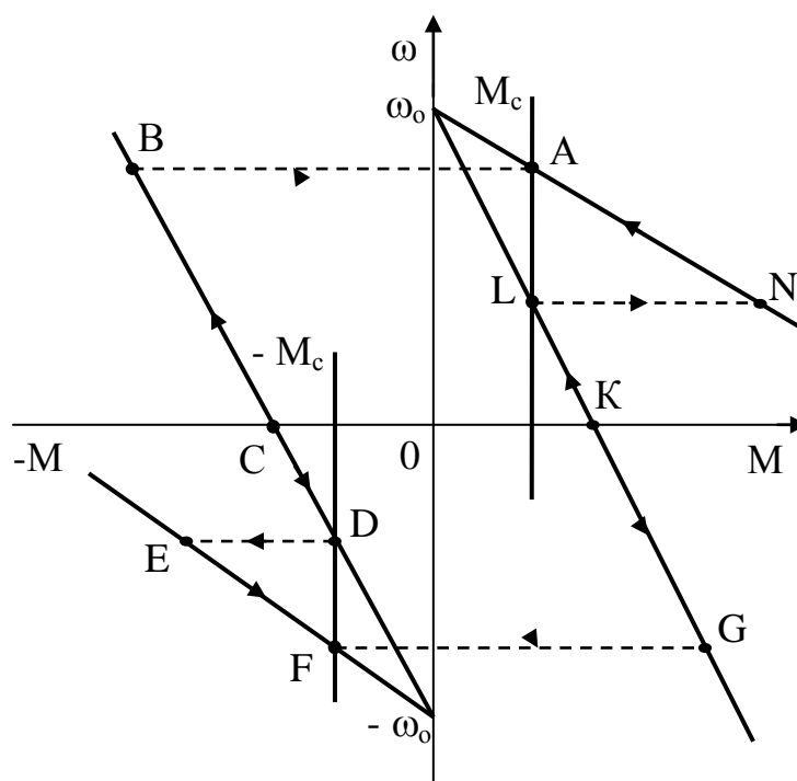
Рисунок 2.25 – Механические характеристики ДПТ НВ в режиме противовключения
