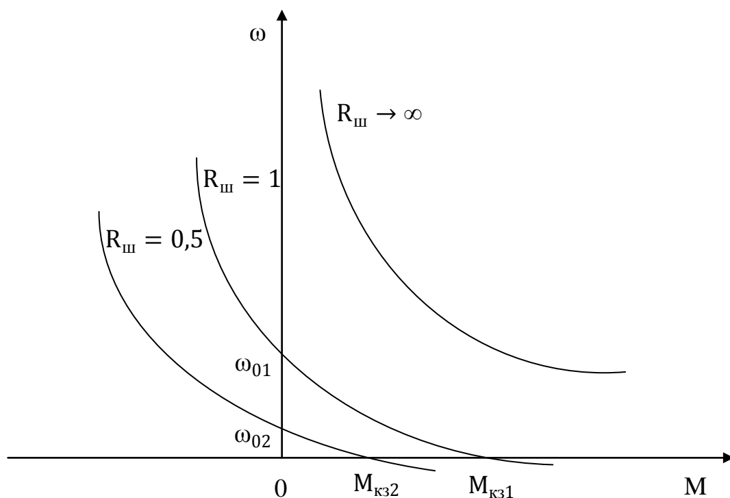
Рисунок 2.15 – Механические характеристики ДПТ ПВ с шунтирующим якорь резистором
